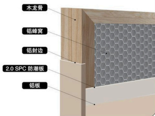
全铝门扇 (2.0 SPC+ 铝面) 木龙骨
