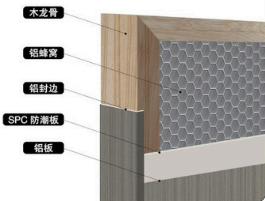
全铝门扇 (4.0 SPC+ 铝面) 木龙骨
